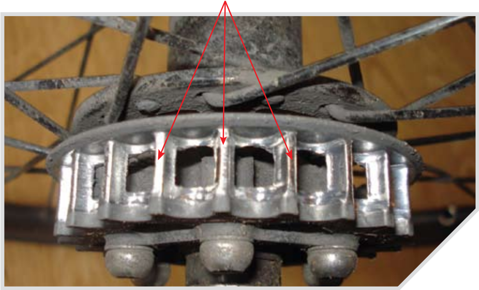
Verschleiß an den Zähnen des CDC-Zahnkranzes
